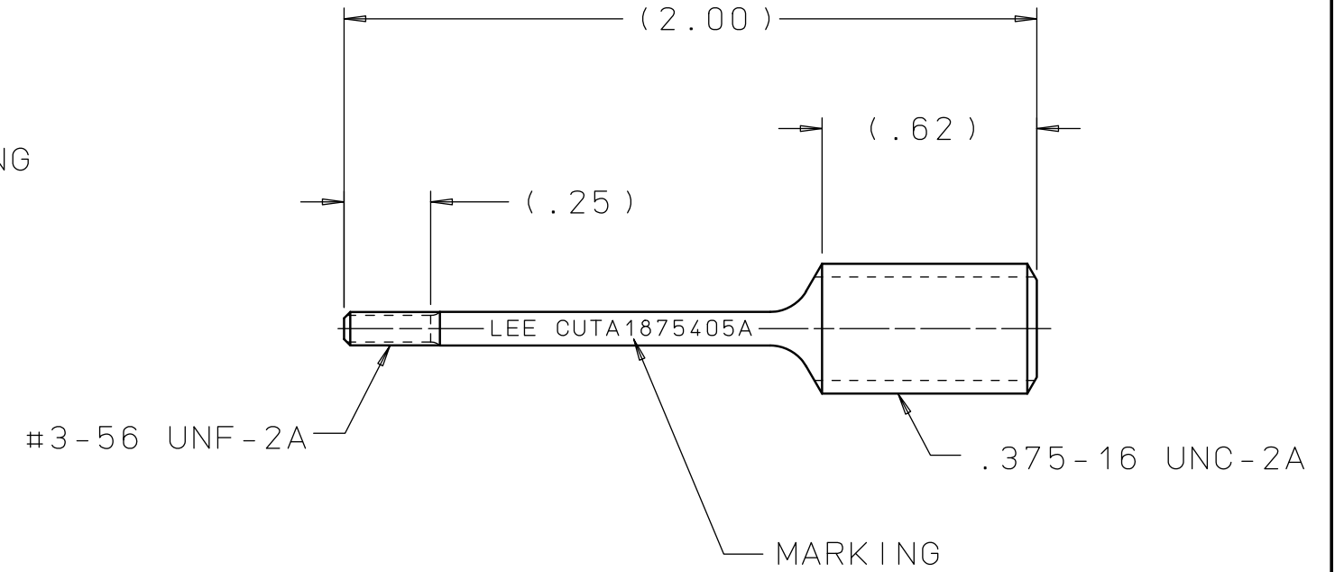
STUD CUTA 1875405A
