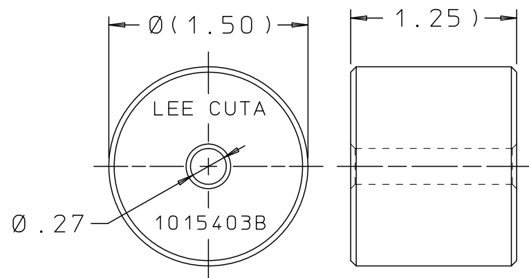
STRIKER, PIN
