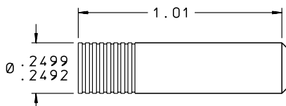
INSERT
