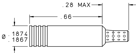
INSERT
