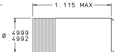
INSERT
